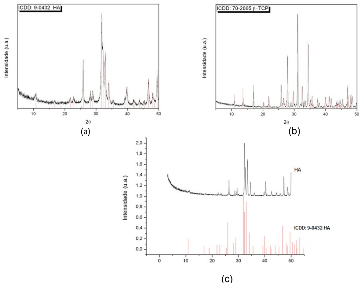
Fig. 2: Difratomogramas dos pós de partida (a) hidroxiapatita, (b) beta-TCP e (c) da amostra sinterizada de hidroxiapatita.
