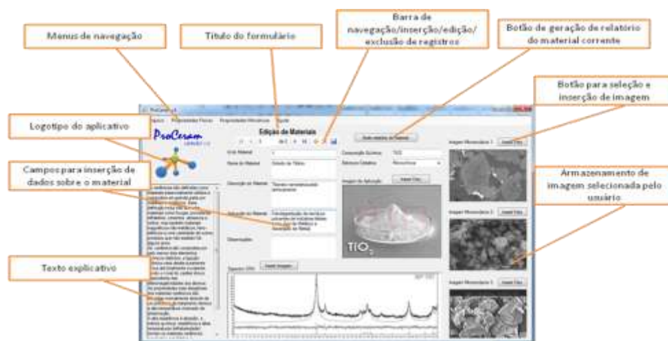
Figura 2 – Representação do formulário de cadastro de materiais - ProCeram
