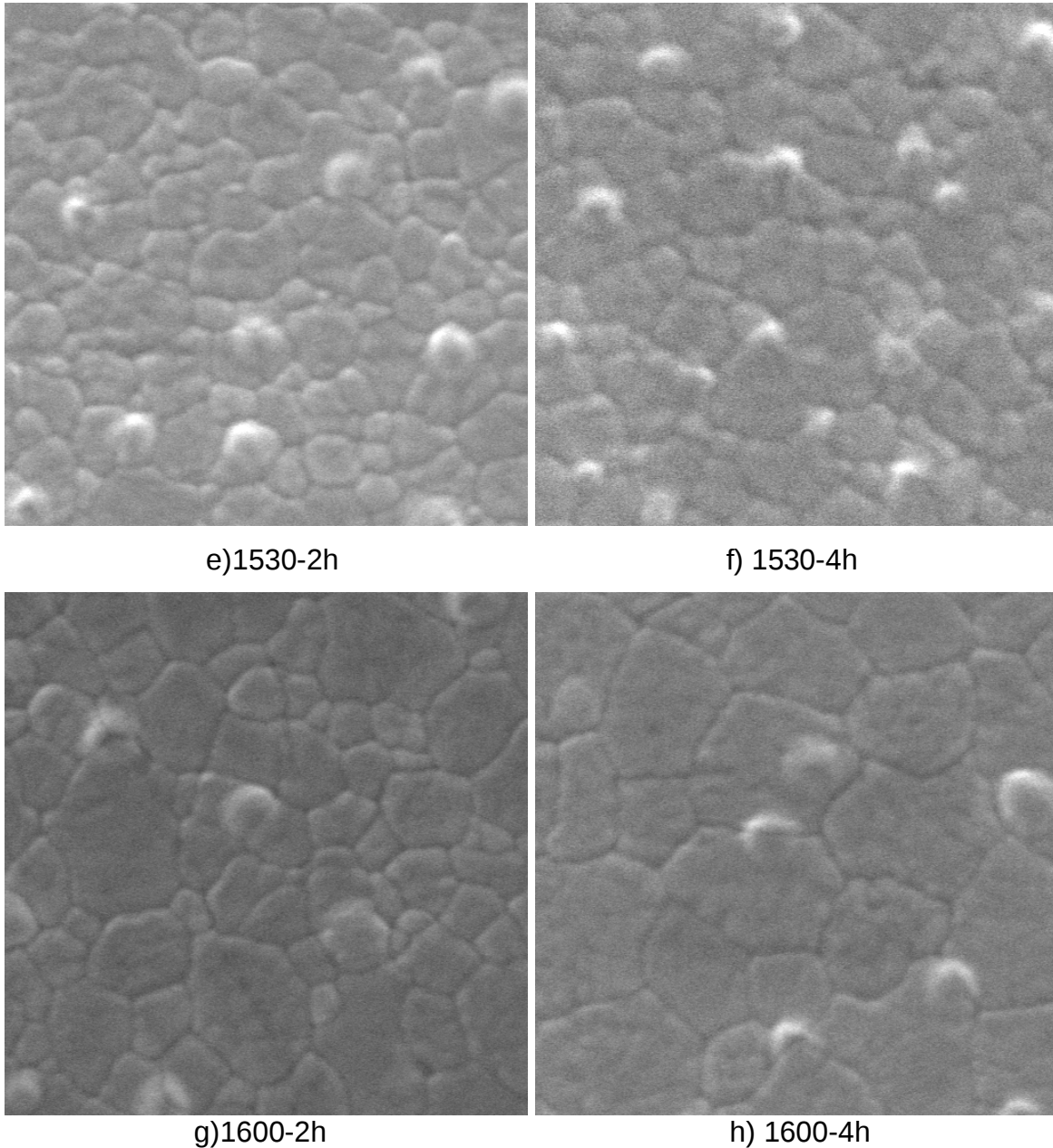
Figura 3. Micrografias obtidas por MEV que revelam a microestrutura de cerâmicas a base de \text{ZrO}_2(3\%\text{Y}_2\text{O}_3) sinterizadas em diferentes condições.
