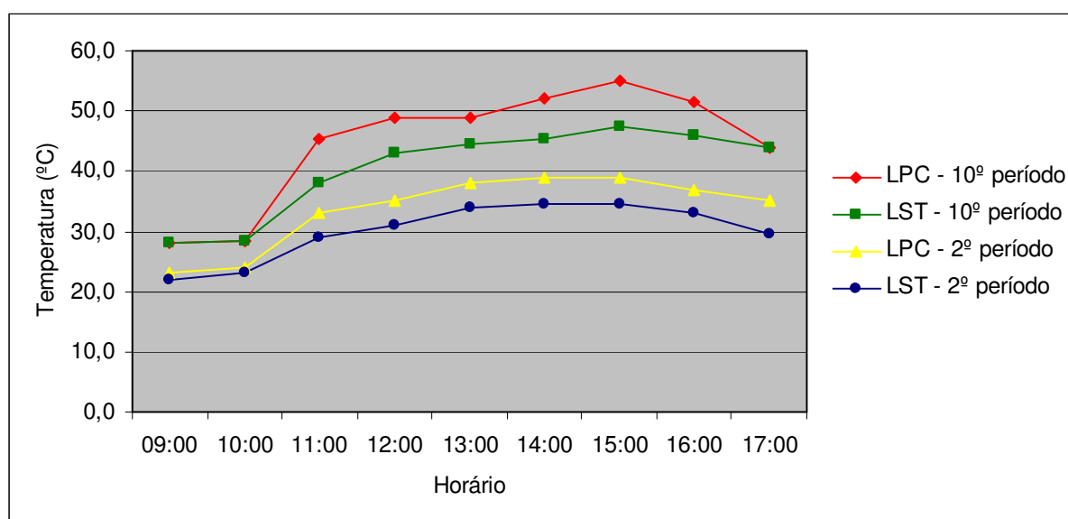
Figura 5 - Temperaturas do lodo nos leitos no 2º e 10º períodos.
