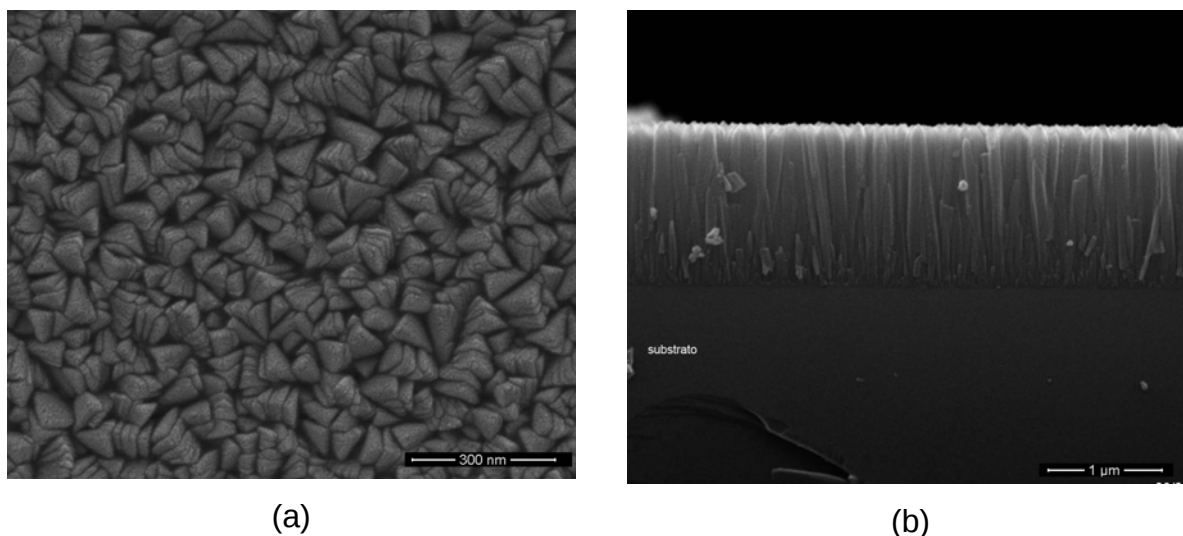
Figura 6: Filme obtido após 1h a 500°C, 50 mbar. Fluxo de N 2 de arraste = 0,3 slm (a) superfície; (b) secção transversal.
