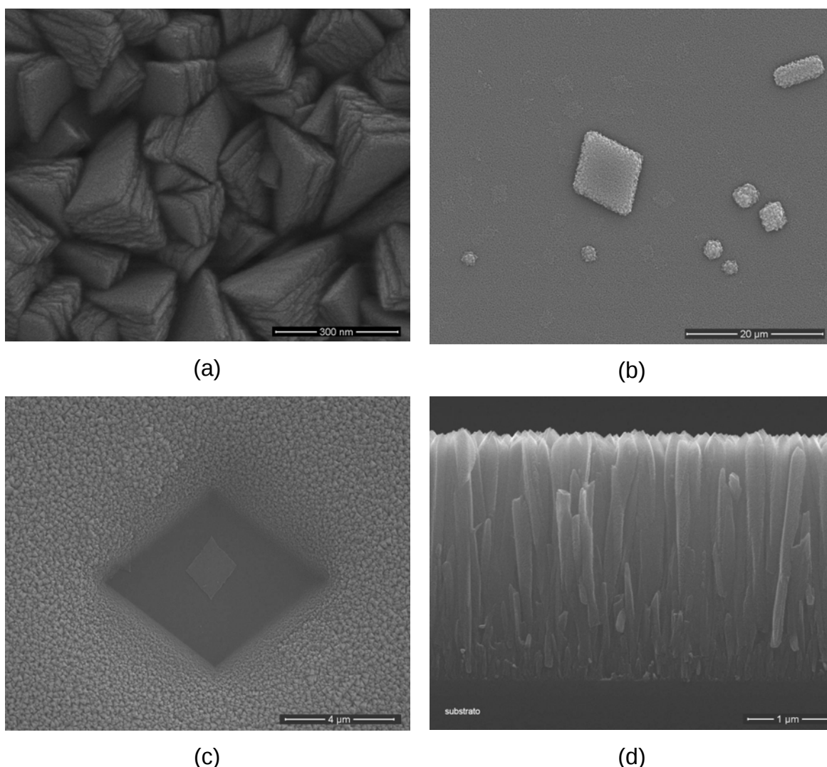
Figura 5: Filme obtido após 1h de crescimento a 500°C, 50 mbar. Fluxo de N_2 vetor = 0 (a) superfície; (b) superfície mostrando partículas destacadas; (c) cavidades resultantes de partículas destacadas; (d) secção transversal.
