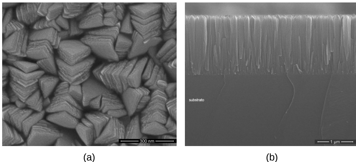
Figura 7: Filme obtido após 1h de crescimento a 500°C, 50 mbar. Fluxo do N 2 vetor = 0,8 slm. (a) superfície; (b) secção transversal.
