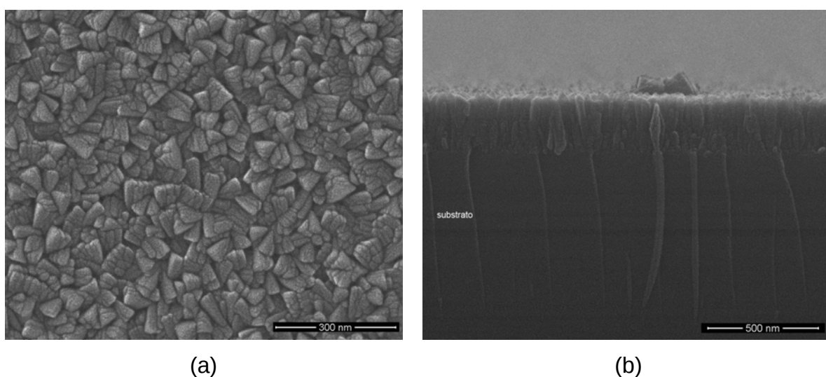
Figura 8: Filme obtido após 15 min de crescimento a 500°C, 50 mbar. Temperatura da fonte = 35°C. (a) superfície; (b) secção transversal.
